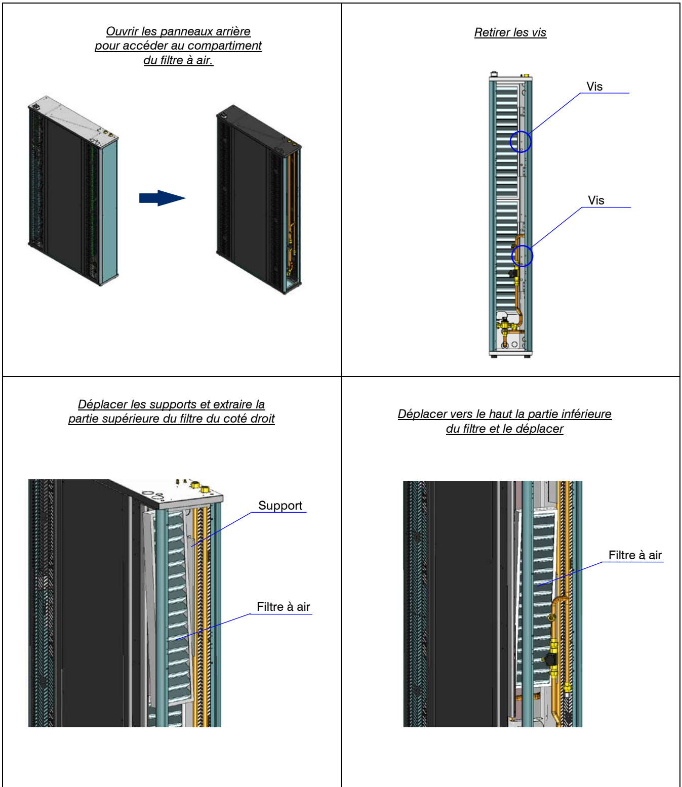
Fig. 13 Contrôle filtre à air
