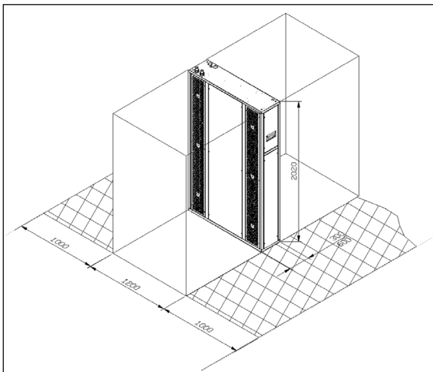
Fig. 7 Zone de service
