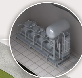
Centrale de compression MOPSH 22 > 385 kW
