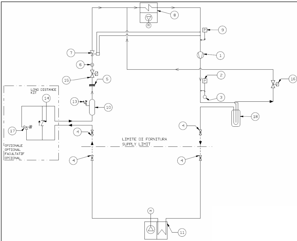
Fig. 3 Circuito frigorifero base
