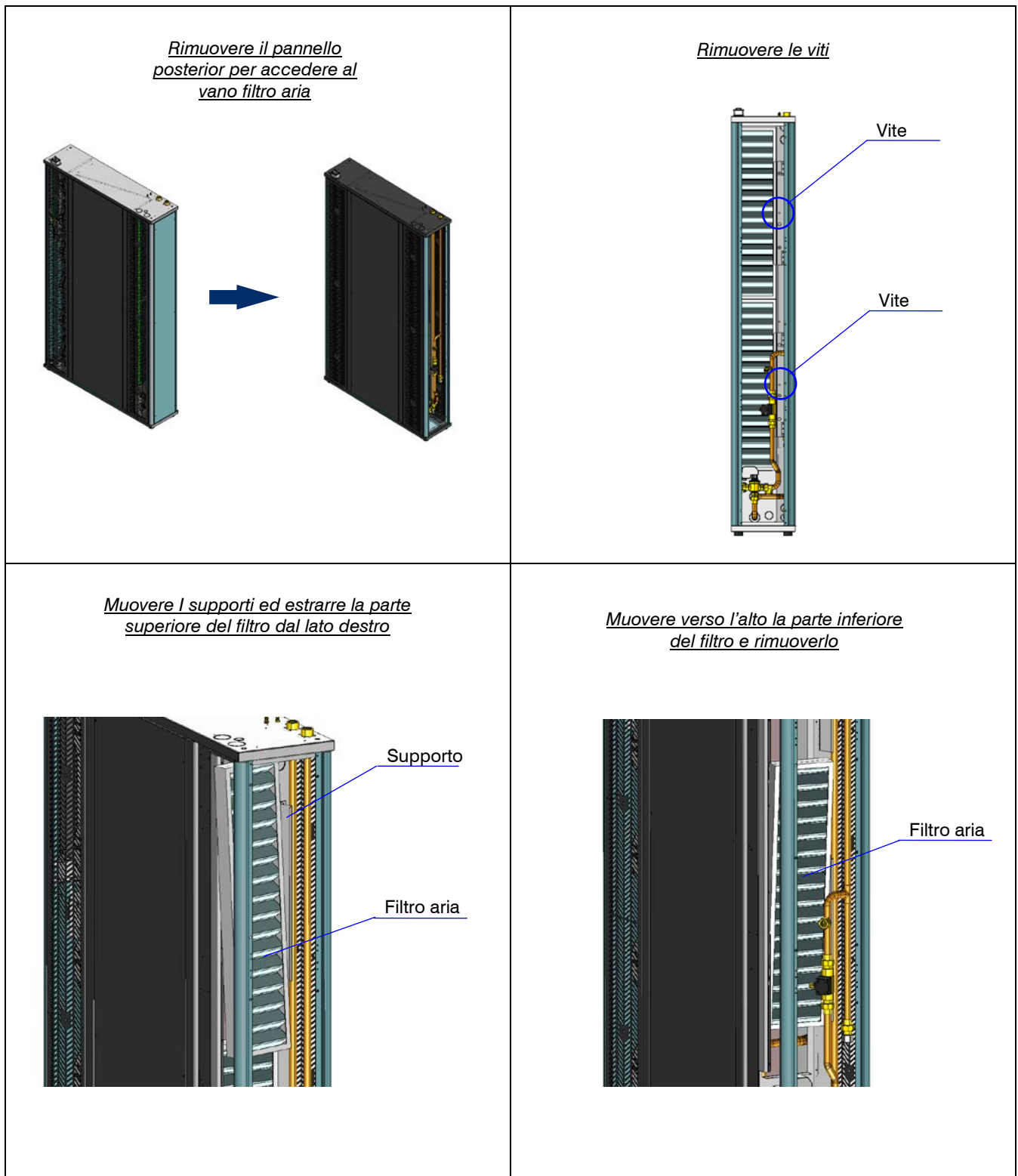
Fig. 13 Ispezione filtro aria
