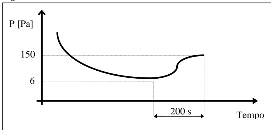
Fig. 9 Ciclo di vuoto
