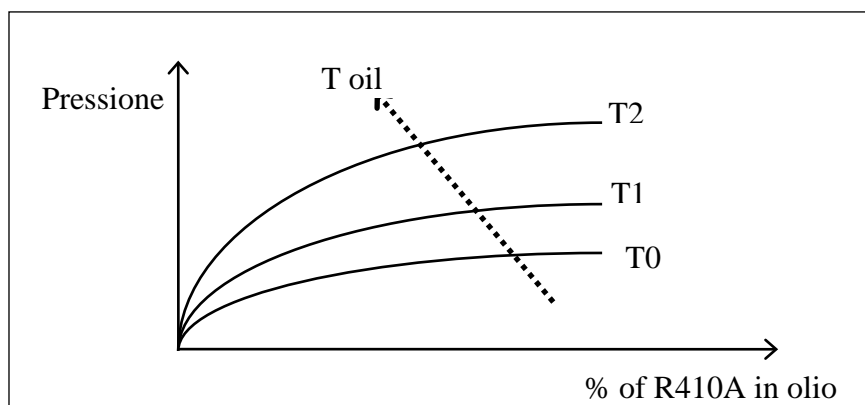
Fig. 12 Grafico legge di Charles
