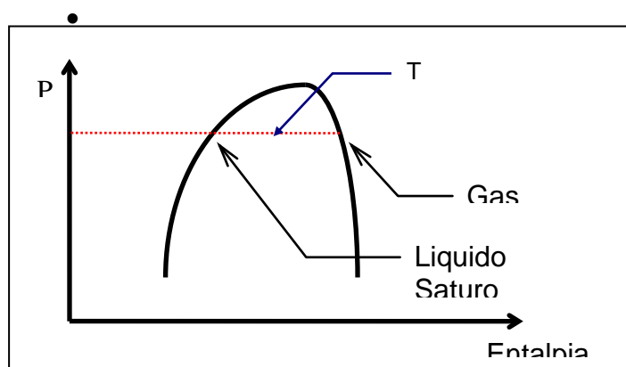
Fig. 8 Diagramma Legge di Gibbs
