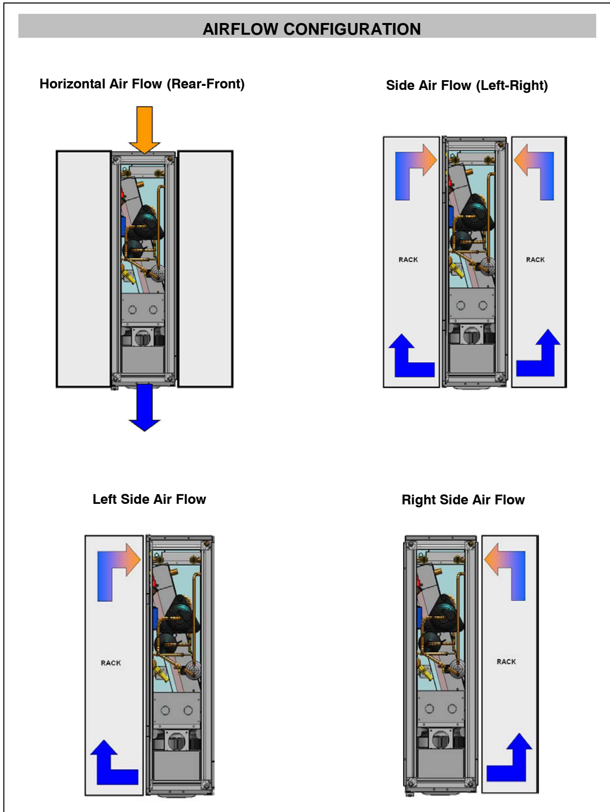
Fig. 11 Schemi funzionali della macchina
